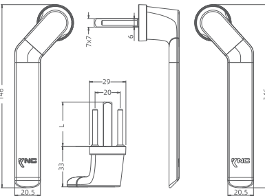
Curved Mini-Rose Spindle Handle (Anodized) 弯柄无基座执手(氧化) 产品编码: KN218MQ | KN218MR 执手高度: 33mm | 33mm 左右规格: 左弯 | 右弯 表面处理: 阳极氧化 方轴规格: 7X7-25/35/40/45/50/68mm
