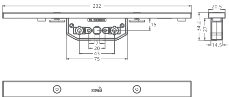
One-Way Drive Gear 单向传动锁盒 产品编码: KN230BN 材料处理: 锌合金 (电镀锌镍) + 铝合金 (氧化) 中 心 距: 15mm 产品规格: 单向传动36mm行程
