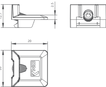
Standard Keeper 锁座（C槽） 产品编码：KN100PL 材料处理：锌合金 锁钉配套：KN100LE、KN100MM、KN100LW、KN100OU、KN100UO、KN100KS-A/B、KN100LI、KN100UP、KN100KQ-A/B
