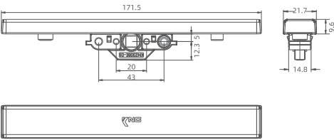
One-Way Drive Gear 单向传动锁盒 产品编码: KN230BE 材料处理: 锌合金 (电镀锌镍) + 铝合金 (氧化) 中 心 距: 5mm 产品规格: 单向传动36mm行程
