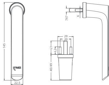
Mini-Rose Spindle Handle 直柄无基座方轴执手 产品编码: KN218LV | KN218MJ 执手高度: 49mm | 40mm 左右规格: 不分左右 表面处理: 粉末喷涂 方轴规格: 7X7-25/35/40/45/50/68mm
