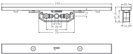
One-Way Drive Gear 单向传动锁盒 产品编码: KN230AW 材料处理: 锌合金 (电镀锌镍) + 铝合金 (氧化) 中 心 距: 12mm 产品规格: 单向传动36mm行程
