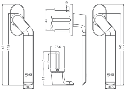
Curved Mini-Base Spindle Handle 弯柄有基座执手 产品编码: KN218MC | KN218MD 执手高度: 33mm | 33mm 左右规格: 左弯 | 右弯 表面处理: 粉末喷涂 方轴规格: 7X7-25/35/40/45/50/68mm
