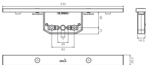
One-Way Drive Gear 单向传动锁盒 产品编码: KN230BL 材料处理: 锌合金 (电镀锌镍) + 铝合金 (氧化) 中 心 距: 30mm 产品规格: 单向传动36mm行程
