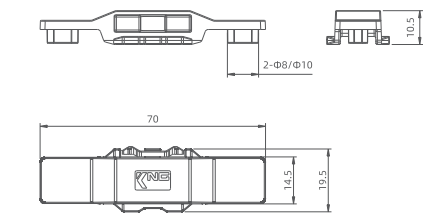
Fork Handle Connector 拨叉连接块 产品编码：KN100KR 材料处理：锌合金 (电镀锌镍) 适用场景：拨叉执手
