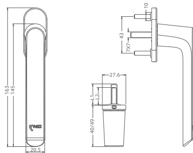
Mini-Base Spindle Handle 直柄有基座方轴执手 产品编码: KN218LS | KN218ML 执手高度: 49mm | 40mm 左右规格: 不分左右 表面处理: 粉末喷涂 方轴规格: 7X7-25/35/40/45/50/68mm
