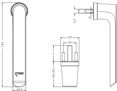
Mini-Rose Spindle Handle (Anodized) 直柄无基座执手(氧化) 产品编码: KN218MZ | KN218MP 执手高度: 49mm | 40mm 左右规格: 不分左右 表面处理: 阳极氧化 方轴规格: 7X7-25/35/40/45/50/68mm
