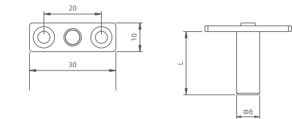
T-Bolt Gear T钉 产品编码：KN100JA 材料处理：304不锈钢 (研磨) 规格长度：22mm/25mm/28mm
