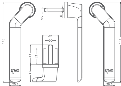
Curved Mini-Rose Spindle Handle 弯柄无基座方轴执手 产品编码: KN218LW | KN218LX 执手高度: 33mm | 33mm 左右规格: 左弯 | 右弯 表面处理: 粉末喷涂 方轴规格: 7X7-25/35/40/45/50/68mm
