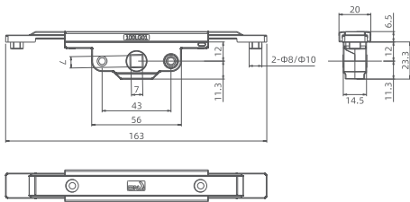
One-Way Drive Gear 单向传动锁盒 产品编码：KN100LG 材料处理：锌合金 (电镀锌镍) 中 心 距：12mm 产品规格：单向传动28mm行程
