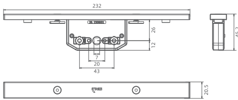
One-Way Drive Gear 单向传动锁盒 产品编码: KN230BJ 材料处理: 锌合金 (电镀锌镍) + 铝合金 (氧化) 中 心 距: 26mm 产品规格: 单向传动36mm行程
