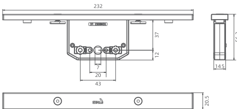
One-Way Drive Gear 单向传动锁盒 产品编码: KN230BK 材料处理: 锌合金 (电镀锌镍) + 铝合金 (氧化) 中 心 距: 37mm 产品规格: 单向传动36mm行程
