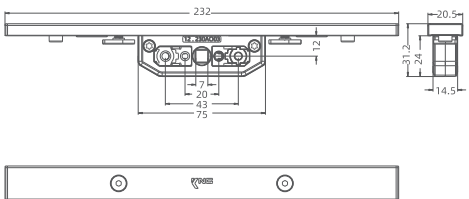
One-Way Drive Gear 单向传动锁盒 产品编码: KN230AO 材料处理: 锌合金 (电镀锌镍) + 铝合金 (氧化) + PA66 中 心 距: 12mm 产品规格: 单向传动36mm行程
