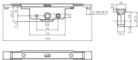
One-Way Drive Gear 单向传动锁盒 产品编码：KN100LH 材料处理：锌合金 (电镀锌镍) 中 心 距：18mm 产品规格：单向传动36mm行程
